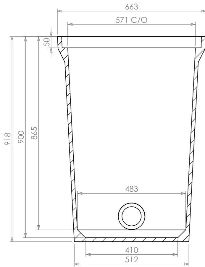
SECTION A-A
